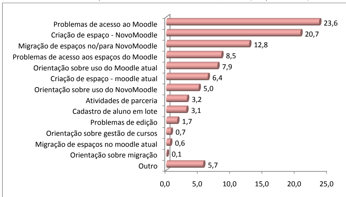
Gráfico 29: Tipos de atividades de atendimento, 2014.2 (em percentuais)
