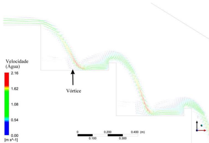
Figura 4 – Campo de velocidade
