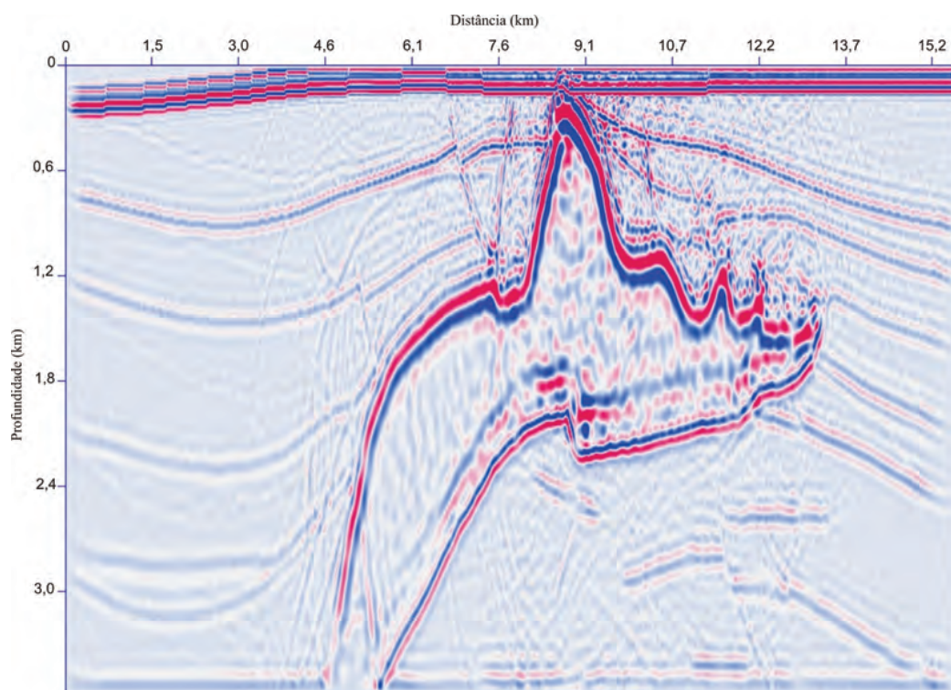
Figura 12 – Resultado da RTM usando FD com 3 termos para os dados do modelo-1 SEG-EAGE reamostrados em 2 ms.
