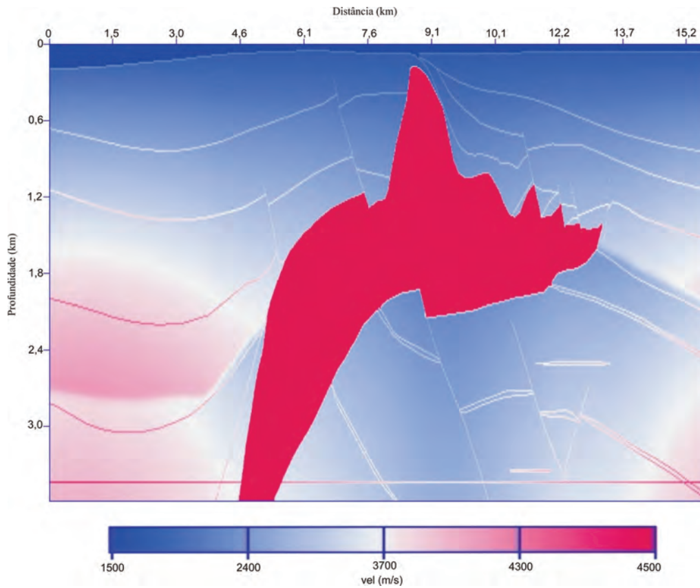
Figura 6 – Campo de velocidade do modelo-1 SEG-EAGE.
