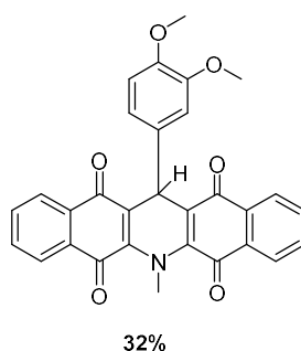
Figura 58: Produto alquilado.
