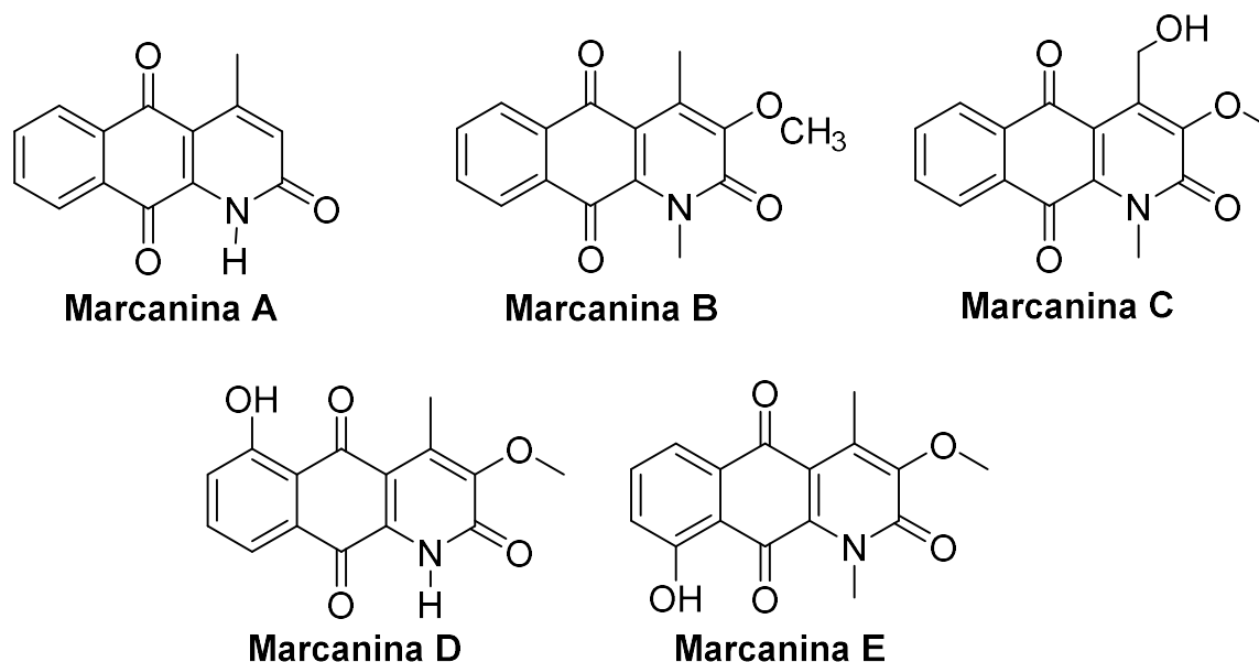
Figura 13: 2-Oxo-aza-antraceno-9,10-dionas naturais.
