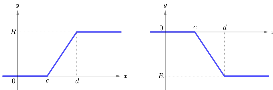
Figura 4 – Protótipos de função rampa
