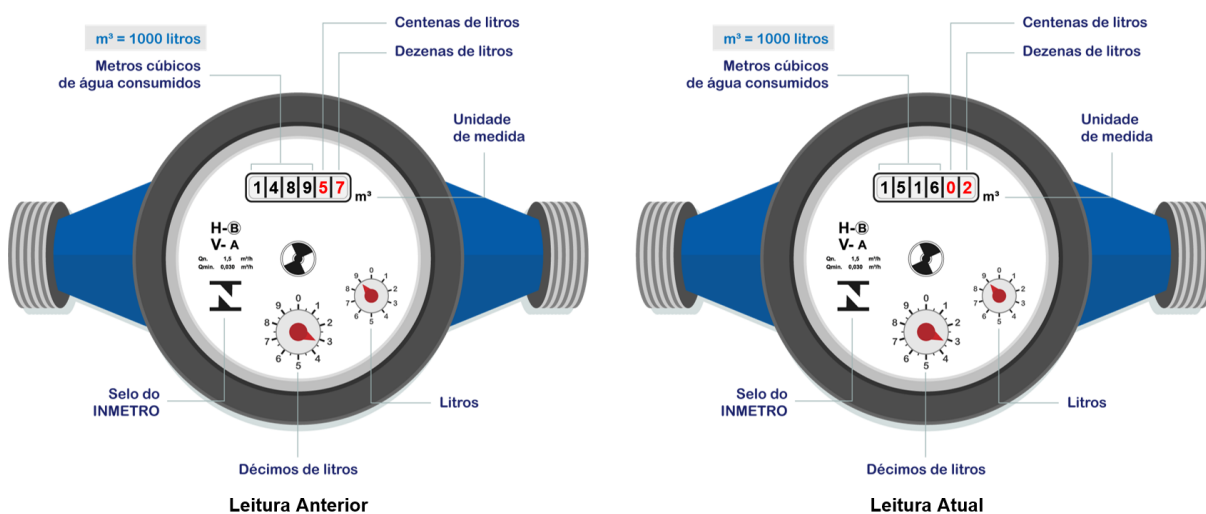
Figura 15 – Leituras anterior e atual de um hidrômetro
