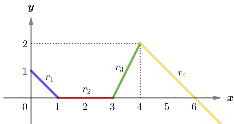
Figura 9 – Exemplo de função poligonal aberta à direita
