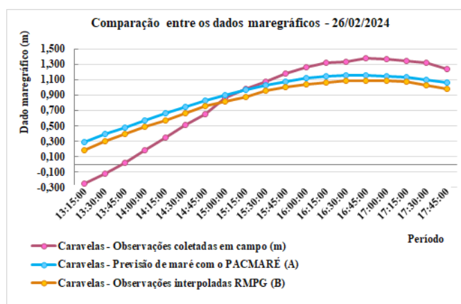
Figura 7 - Comparação entre os dados mareográficos A, B e os dados obtidos em campo em Caravelas. Fonte: Os autores (2024).
