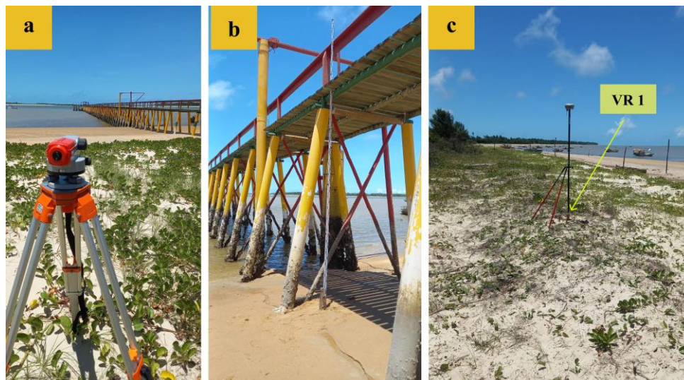
Figura 4 - Coleta dos registros maregráficos em Caravelas/BA: (a) Nível óptico (b) Estação de Observação de Caravelas (EOM) (c) Rastreamento GNSS. Fonte: Os autores (2024).
