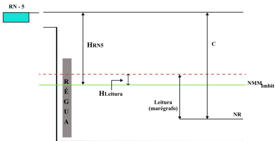
Figura 5 - Diagrama descritivo de uma leitura no marégrafo de Belmonte. Fonte: Os autores (2024).
