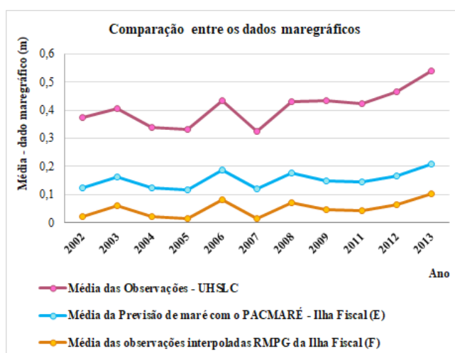
Figura 9 - Comparação entre os dados maregráficos E, F e os dados obtidos por meio do UHSLC. Fonte: Os autores(2024).
